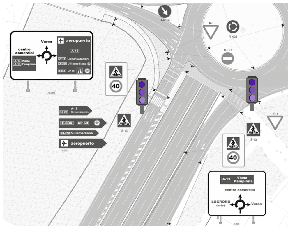
Plano de la actuación.
